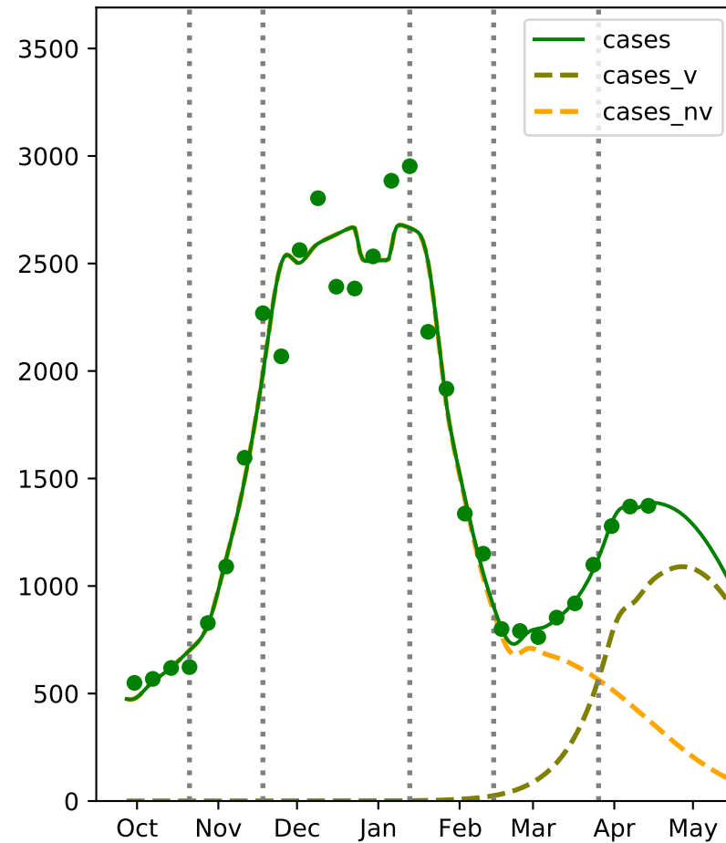
Maryland: April 18 fit
